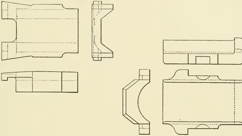
Fig. 18. M. C. B. Journal Bearing and Wedge
